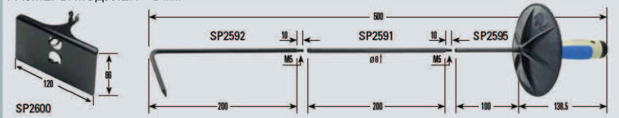
РАЗМЕРЫ МОДУЛЕЙ – в мм
